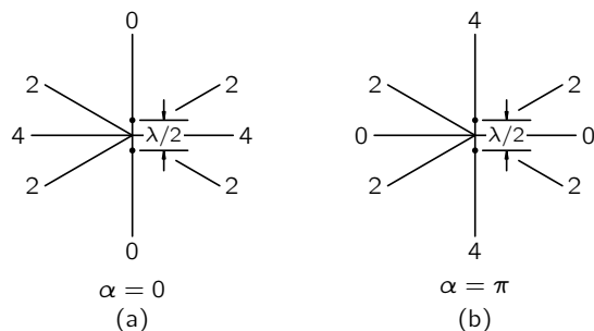
图 29.5: 来自相聚半个波长的两个偶极振子的场在不同方向上的强度 (a) 同相 ( \alpha = 0 ); (b) 相位差半个周期 ( \alpha = \pi )
