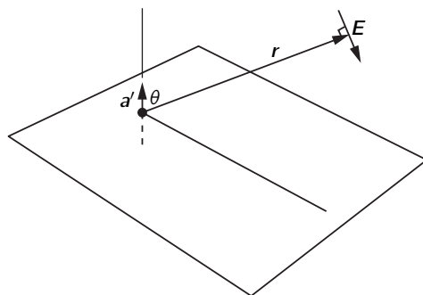
图 29.1: 由推迟加速度为 a' 的正电荷产生的电场 \mathbf{E}
