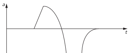
图 29.2: 某电荷的加速度与时间的关系
